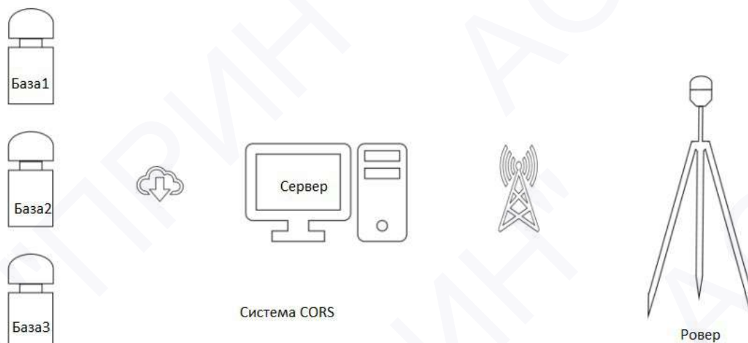
Рис.4.8. Схема работы по протоколу NTRIP от сети базовых станций Для этого режима работы необходима SIM-карта и действующая учётная запись для получения RTK поправок от сети ПДБС. Установите SIM-карту, прежде чем включать приёмник.
