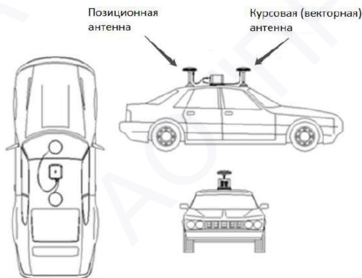
Рис. 3.3. Установка антенн на автомобиле
