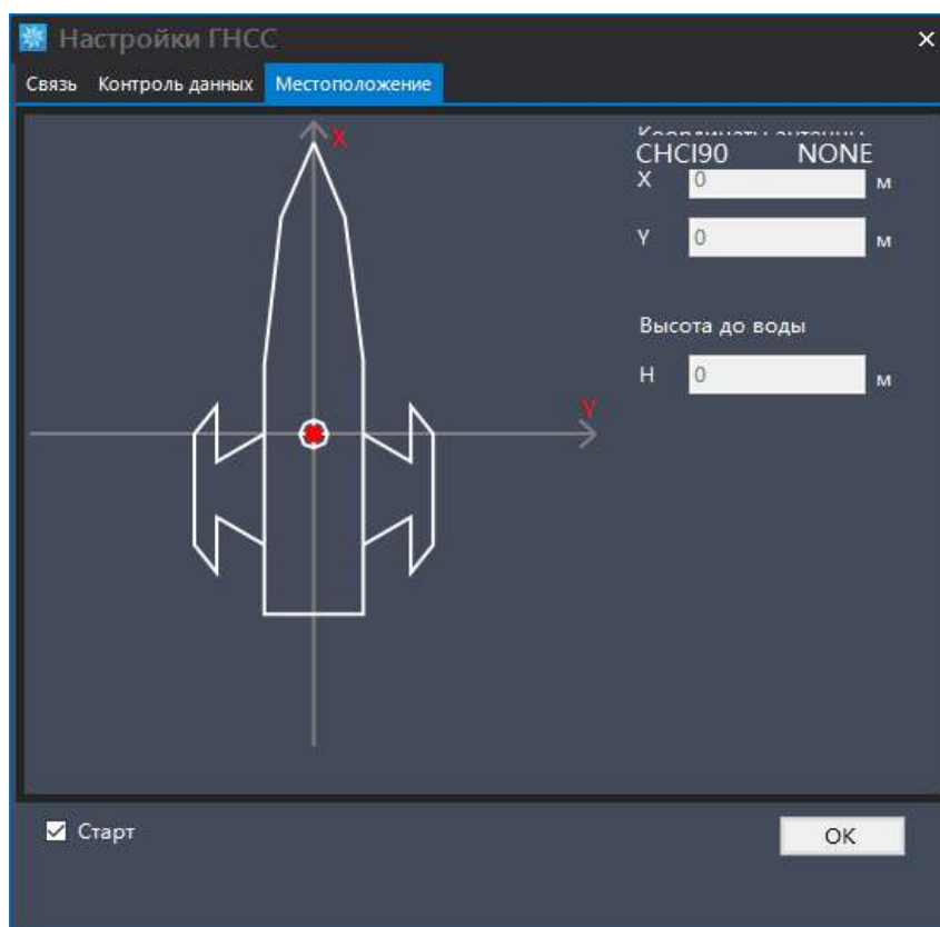
Рис. 4.6 Настройка параметров местоположения ГНСС-приёмника
