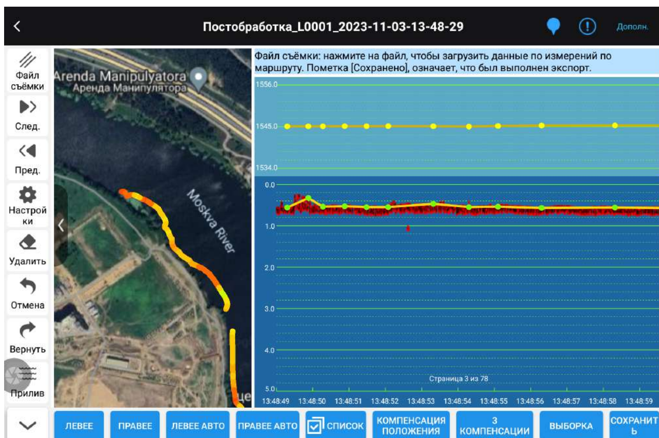
Рис. 5.15 Меню обработки данных
