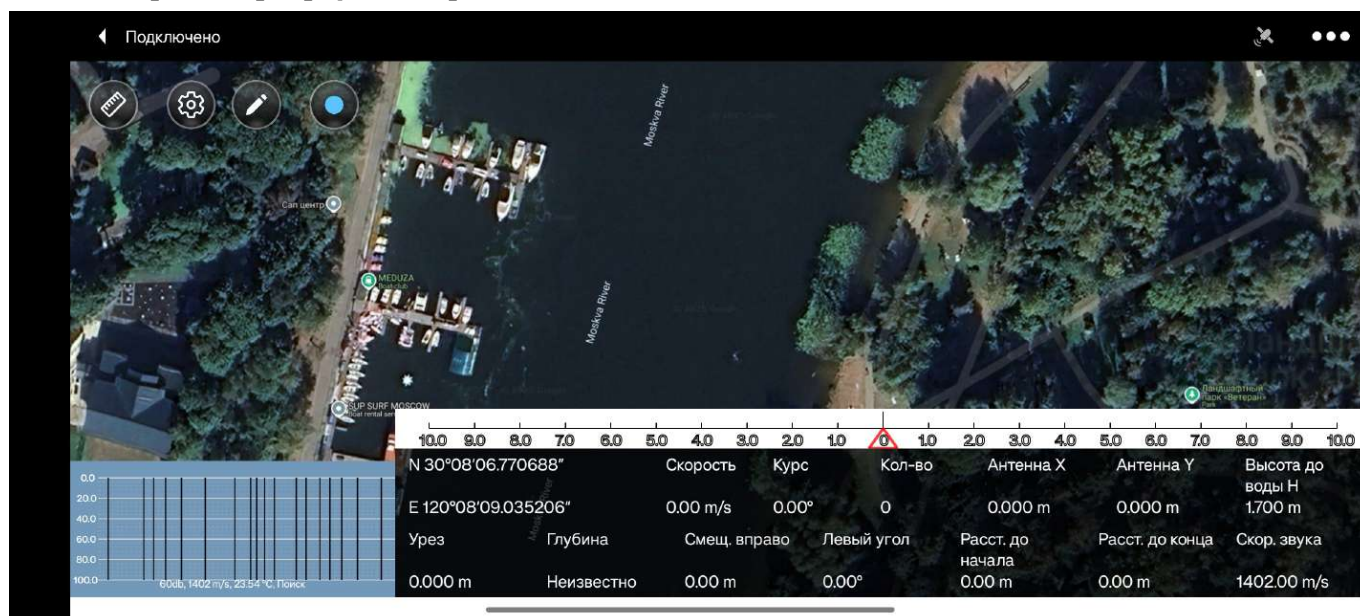
Рис. 5.7 Проект в ПО EasySail
